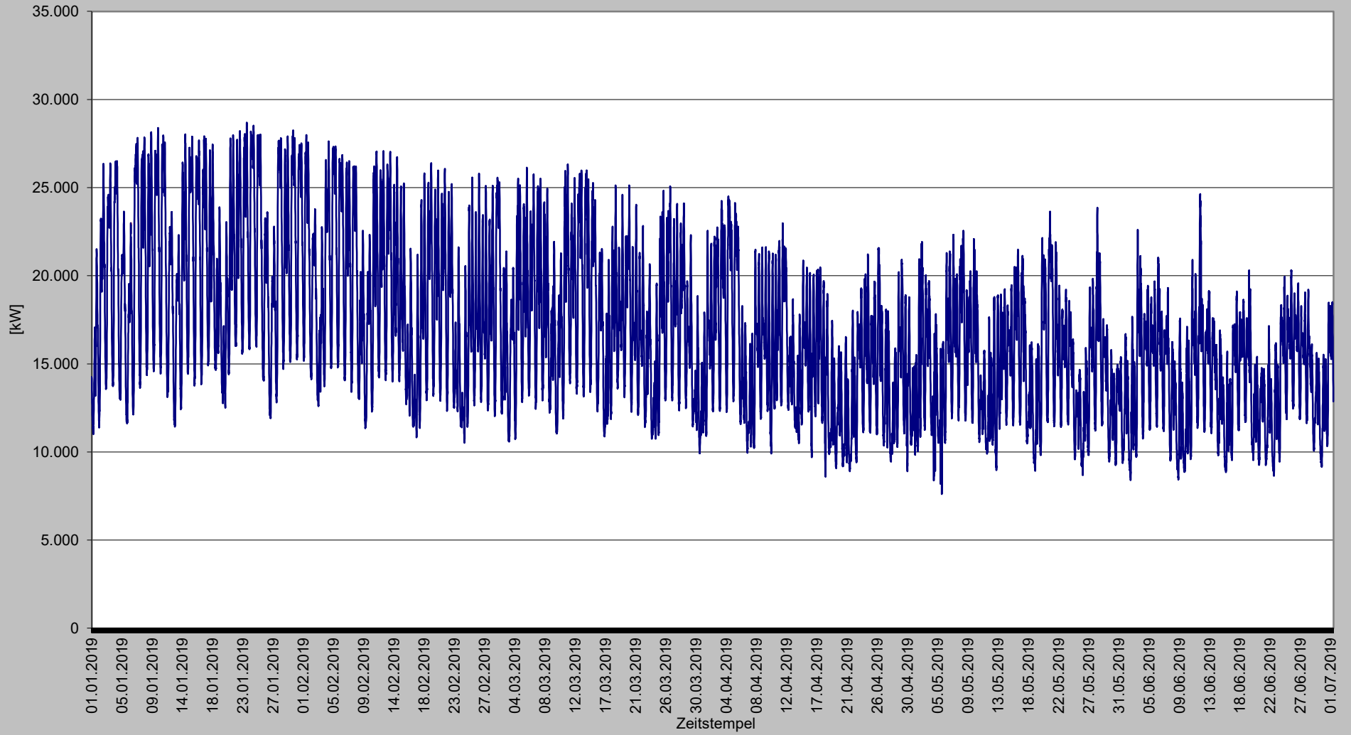
Lastverlauf im Verteilnetzgebiet der Stadtwerke Dülmen GmbH im 1. Halbjahr 2019
