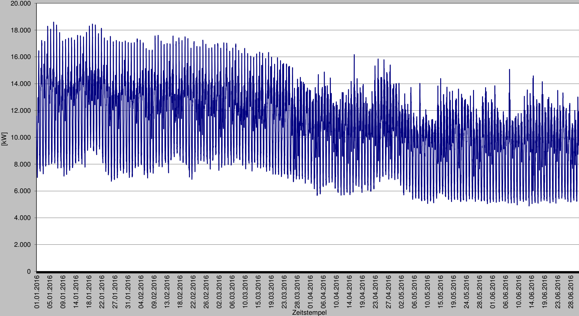
Lastverlauf Nsp. - oL. im Netzgebiet der Stadtwerke Dülmen GmbH für das 1. Halbjahr 2016
