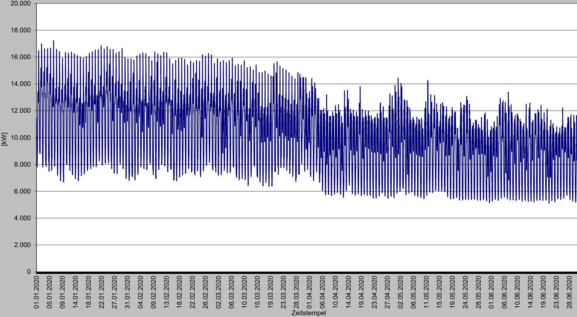
Lastverlauf Nsp. - oL. im Netzgebiet der Stadtwerke Dülmen GmbH für das 1. Halbjahr 2020
